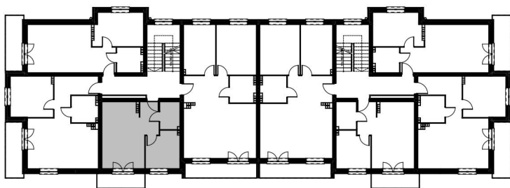
USYTUOWANIE MIESZKANIA RZUT 2-GO PIĘTRA
